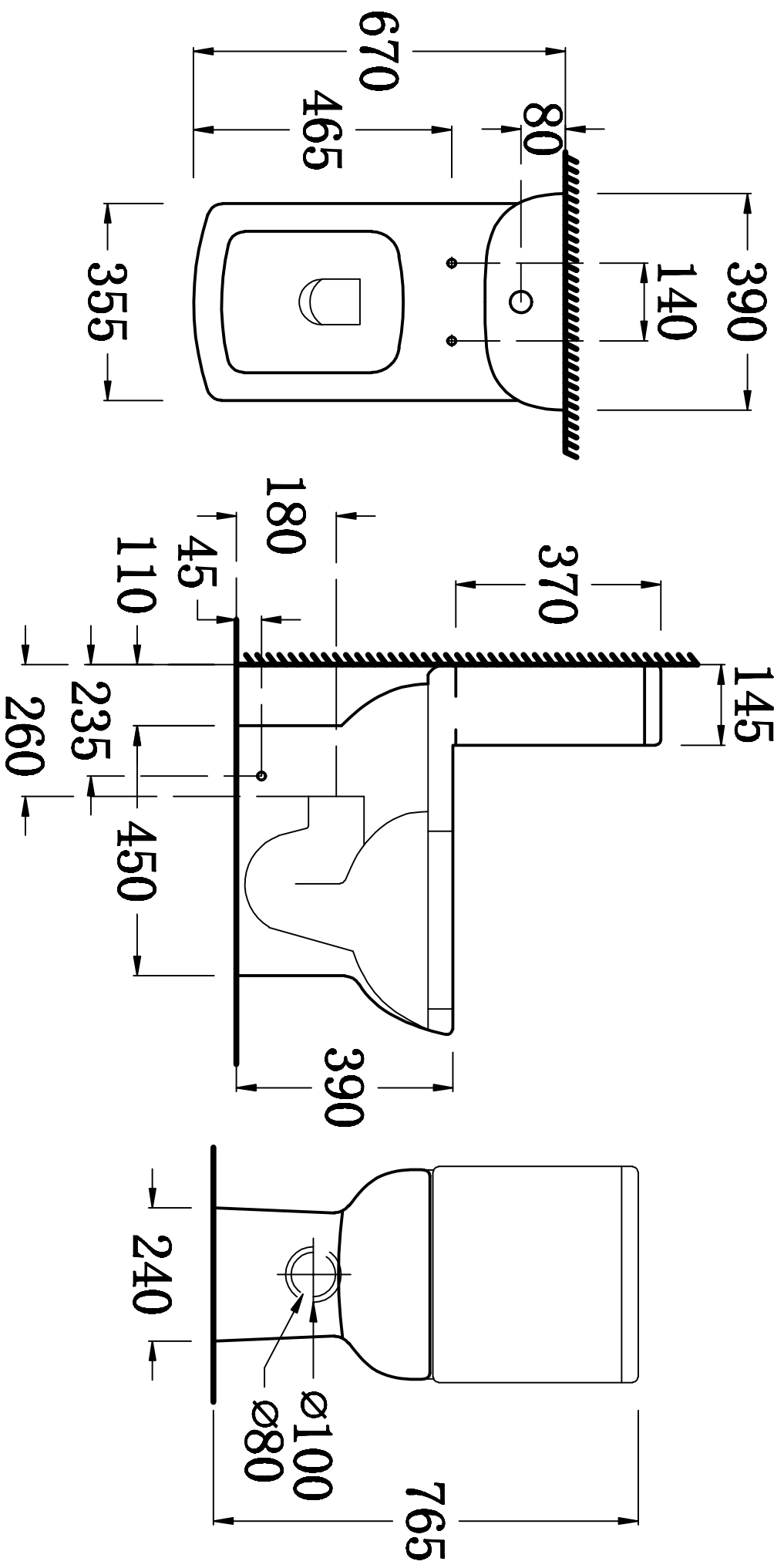
俯视图
